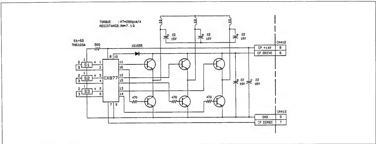
Fig. 4-6-7. Capstan Motor
